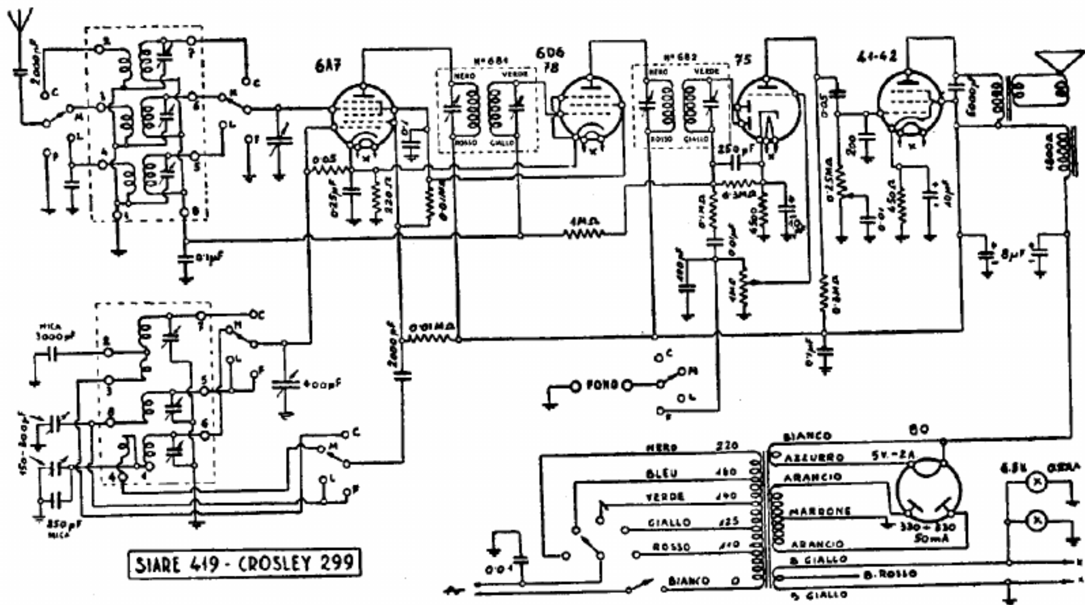
RADIO SIARE — Modelli « Siare 419 » e « Crosley 299 » · Produzione 1937 Media frequenza: 468 kHz.
